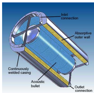
Fan Silencers
